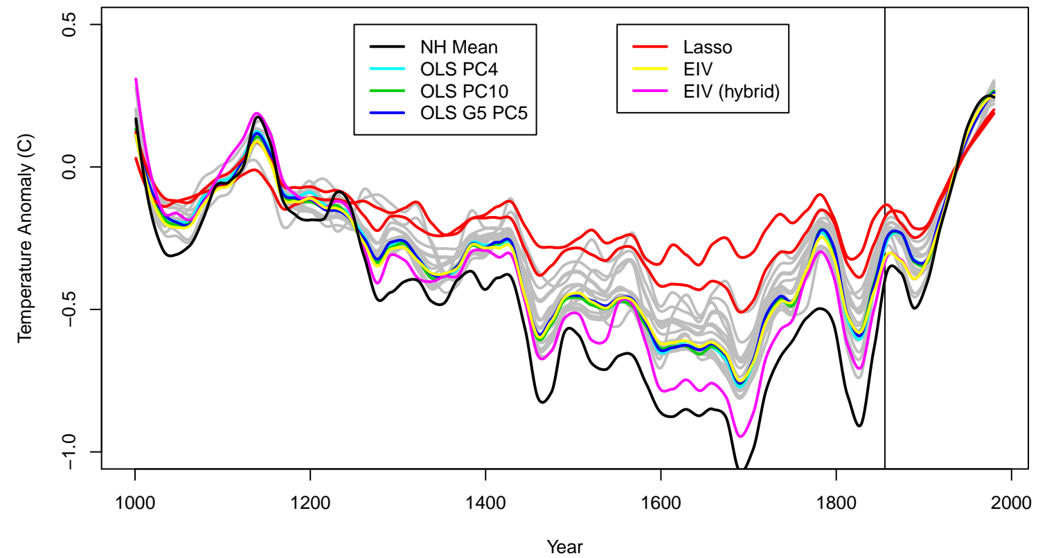
d) Pseudo-proxy test (N=104): GKSS
