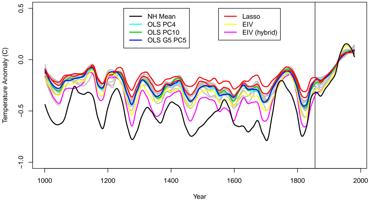
a) Pseudo-proxy test (N=59): CSM
