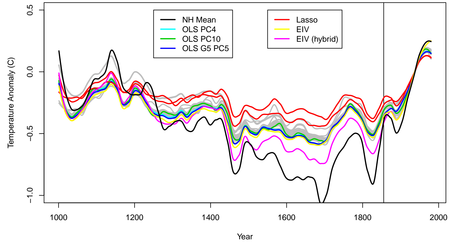
b) Pseudo-proxy test (N=59): GKSS
