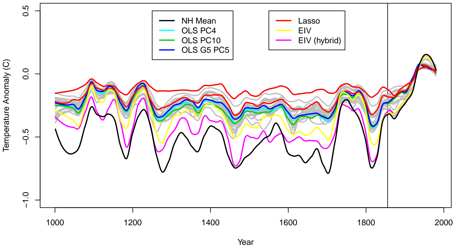
c) Pseudo-proxy test (N=104): CSM
