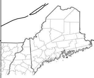
8: BLIZZARD
